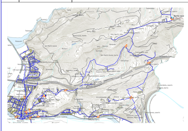
Ubicación de caudalímetros sectoriales existentes
